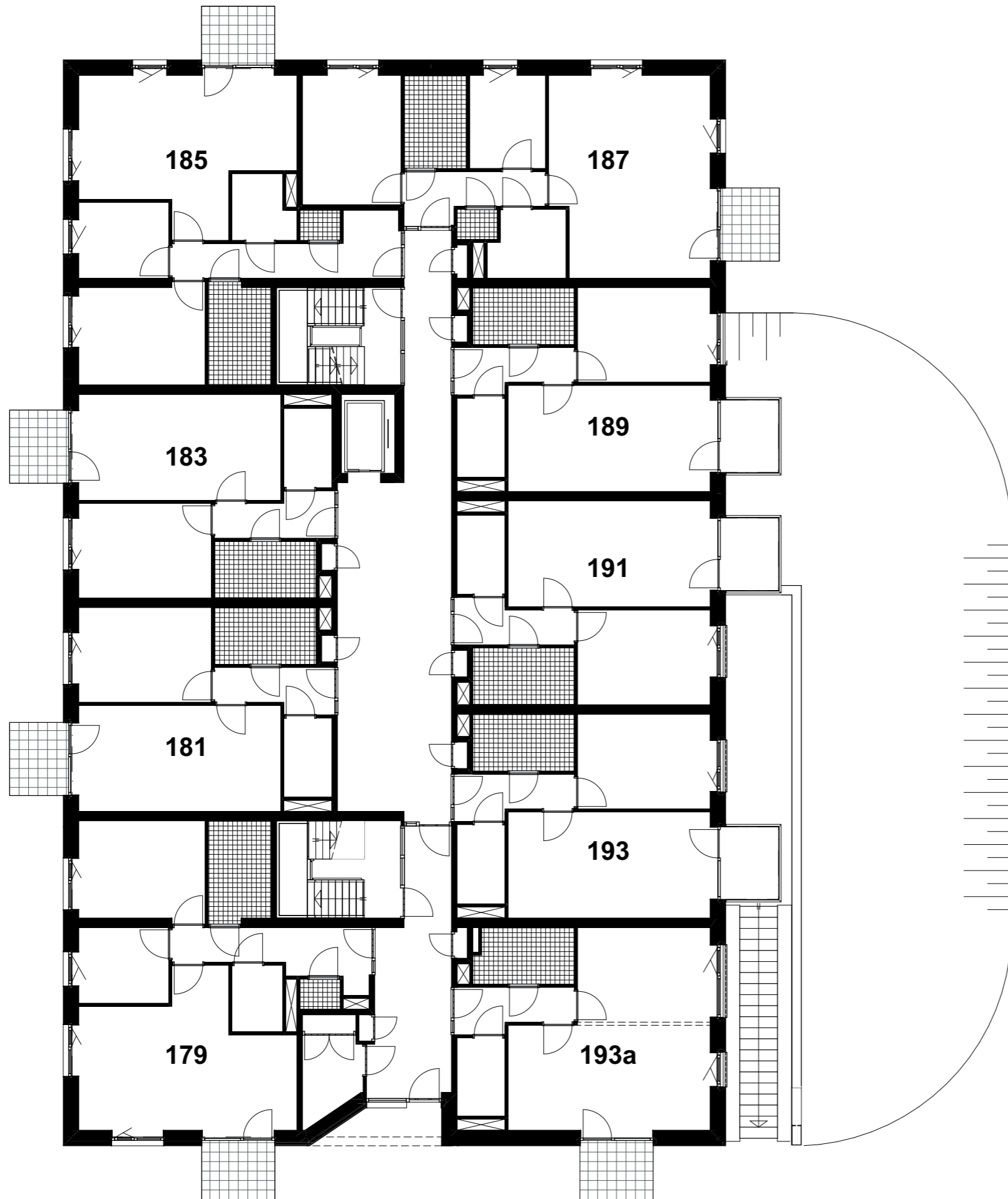
BEGANE GROND schaal 1:150
